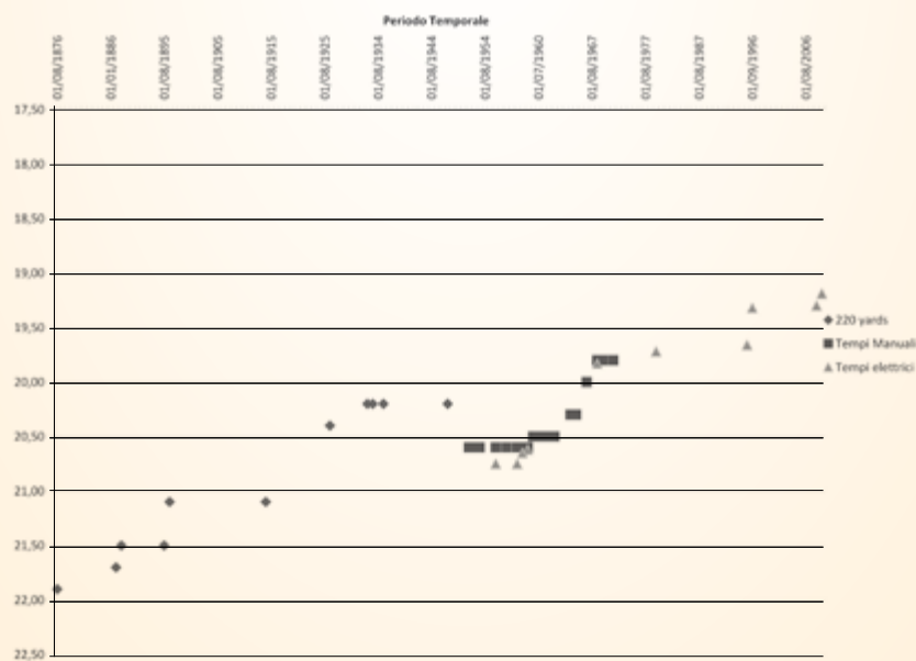
Progressione del record mondiale dei m.200 piani. I rombi si riferiscono ai 200 m in rettilineo; i quadrati ai tempi rilevati con il cronometraggio manuale; i triangoli a quelli rilevati elettronicamente.
